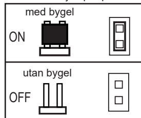
Version med jumper på kretskortet
